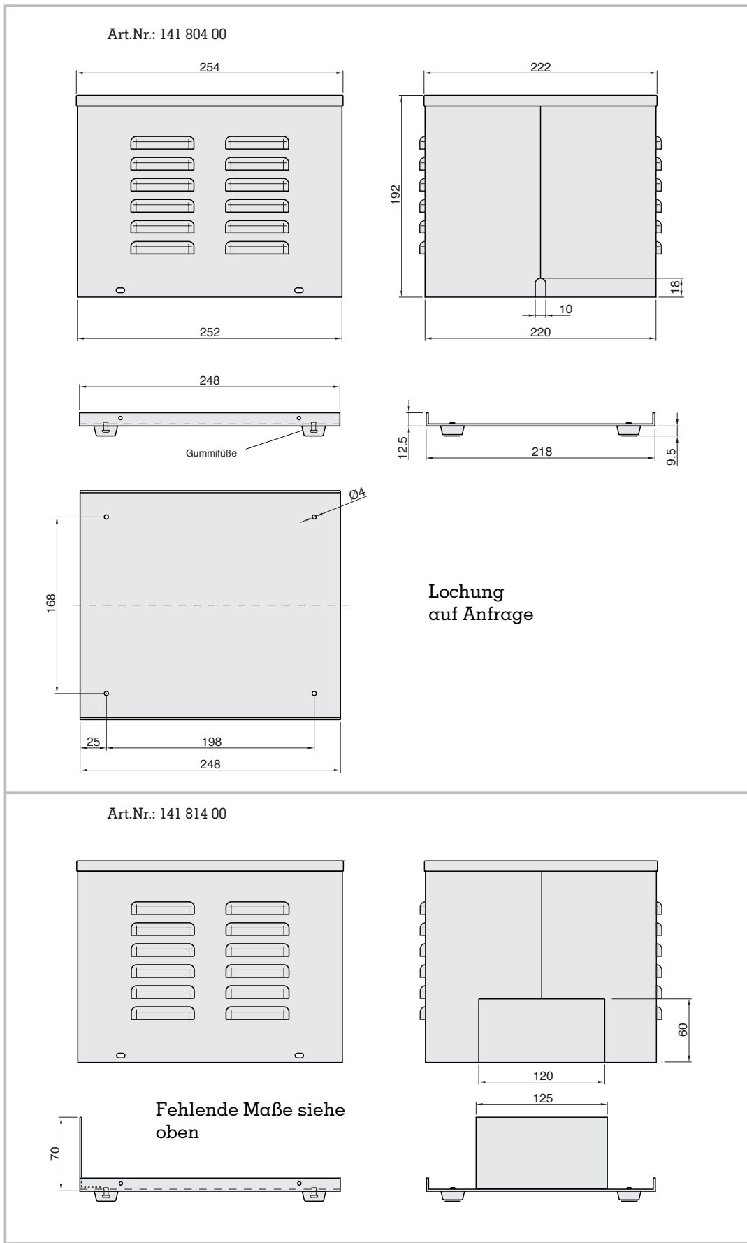
Gehäuse mit Winkel für Kabelverschraubung
